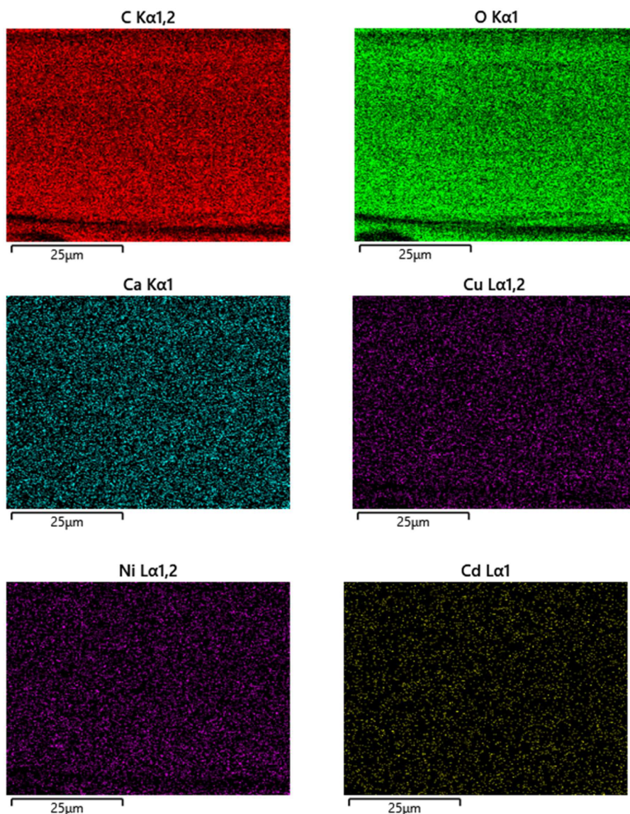
Fig. 10. SEM-EDX mapping of SAlg-MoF (1 %).
