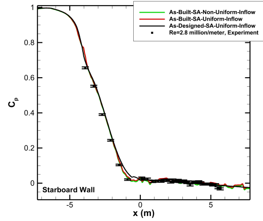
(d) C_p at starboard wall centerline
