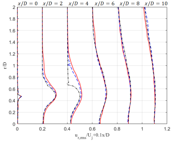
(d) radial velocity fluctuations
