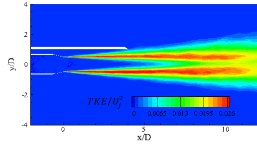
(d) Turbulent kinetic energy in the isolated jet ( H/D=1 )
