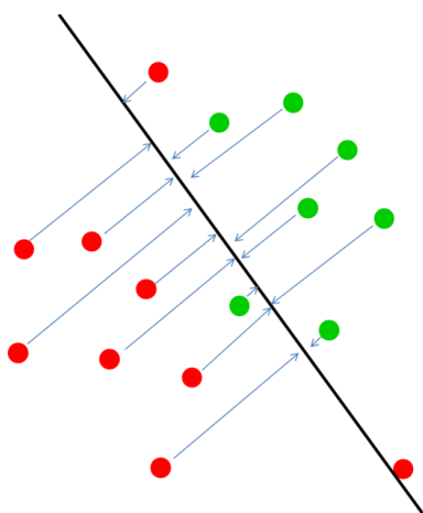
A: Linear Discriminant Analysis (LDA)
