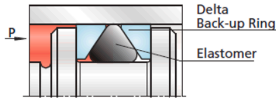
Fig. 2. Turcon® Wedgpak® II Seal [16].
