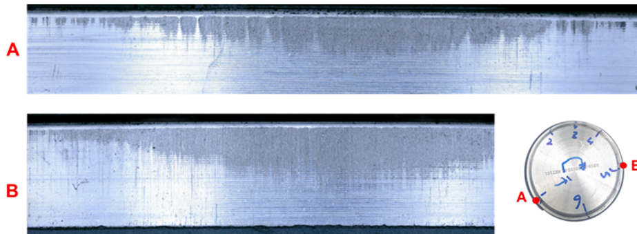
Fig. 20. Piston damage.
