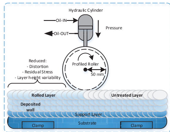
Fig. 2. - WAAM Online Rolling
