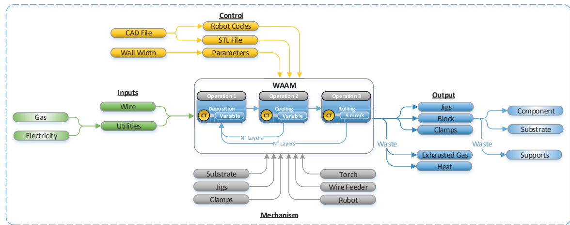
Fig. 3. - WAAM IDEF0
