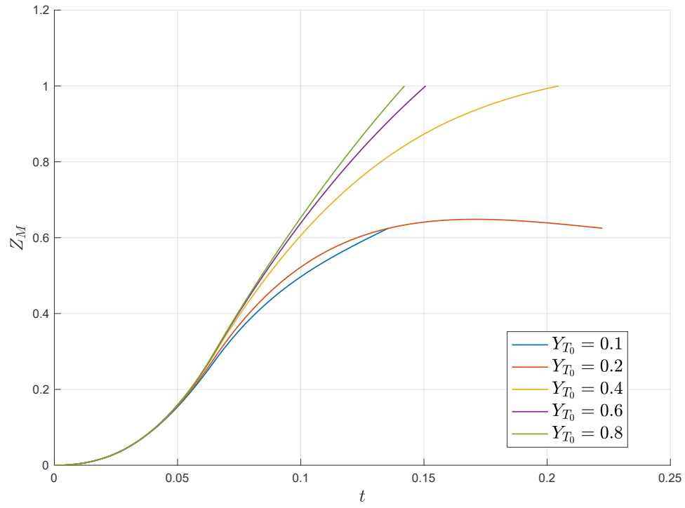
Fig. 22. Case 3. Altitude History for Pure PNG
