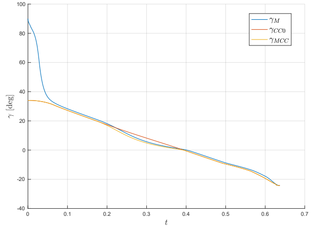
(d) Y_{T_0} = 0.6
