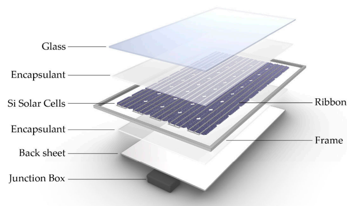
Figure 4. Structure of a PV module [28].
