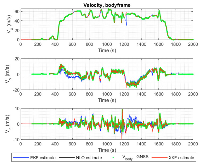
(d) Velocity estimates in body frame.
