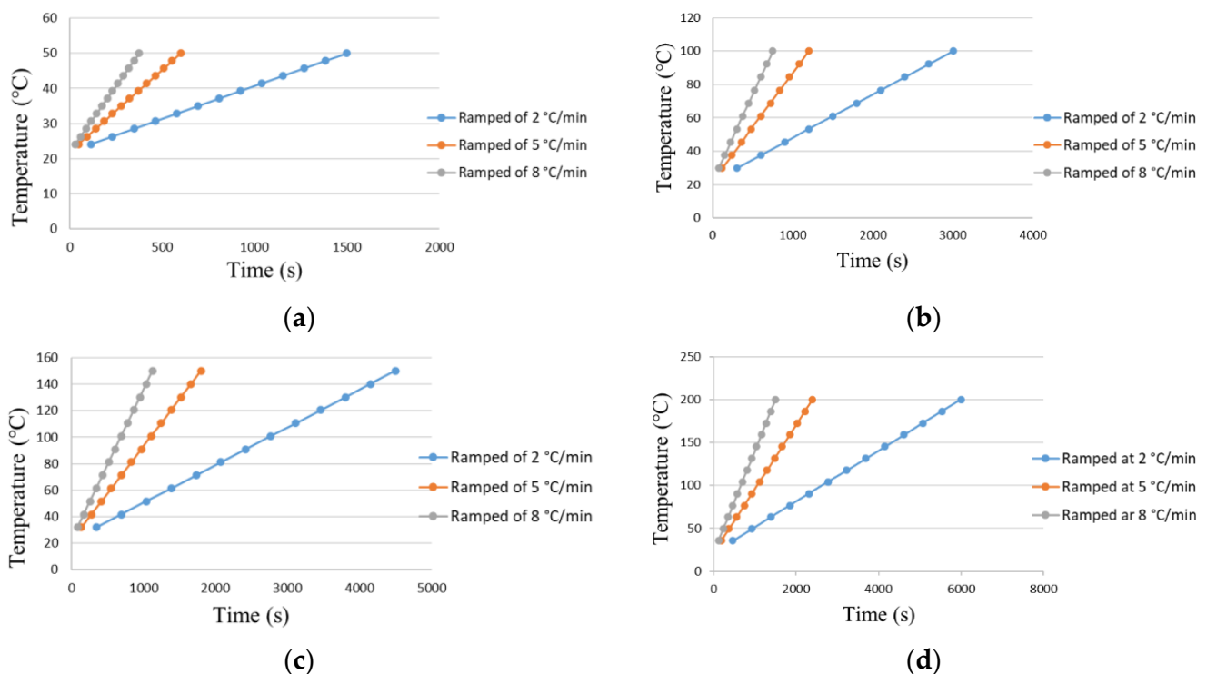
Figure 7. Temperature exposure duration for (a) 50\text{ }^{\circ}\text{C} ; (b) 100\text{ }^{\circ}\text{C} ; (c) 150\text{ }^{\circ}\text{C} ; (d) 200\text{ }^{\circ}\text{C} .
