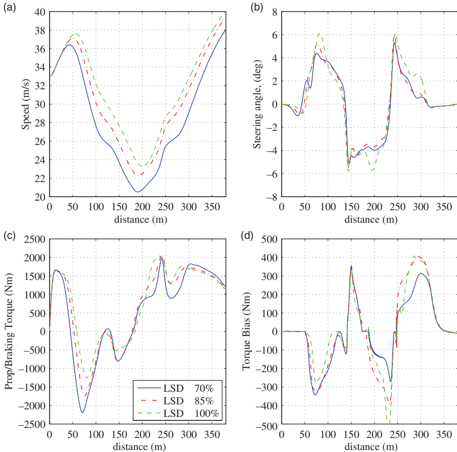
Figure 12. (a) Absolute speed ( \sqrt{U^2 + V^2} ) (b) steering angle, \delta (c) total propulsive/braking torque, \gamma_t (d) optimal torque bias T_b = \frac{1}{2}(T_3 - T_4) .
