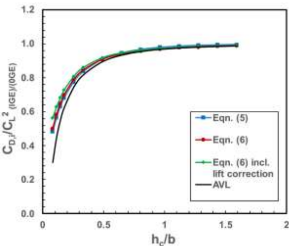
Fig. 8: NACA0012, K_2
