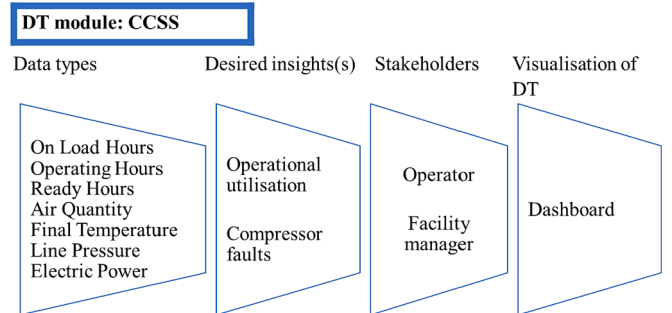
Fig. 9. DT visualisation of the CCSS module.
