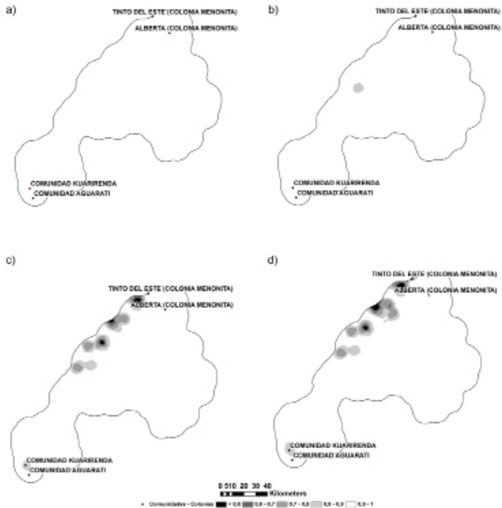
Figura 2. Relación métrica para el porcentaje del paisaje (PLAND) en Baños de Isoso para los años 1986 (a), 1991 (b), 2001 (c) y 2005 (d).
