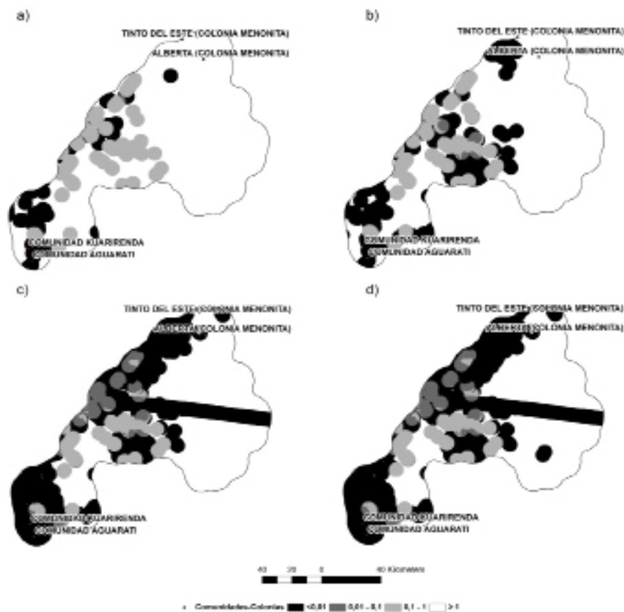
Figura 5. Relación métrica para la densidad de borde (ED) en Baños de Isoso para los años 1986 (a), 1991 (b), 2001 (c) y 2005 (d).
