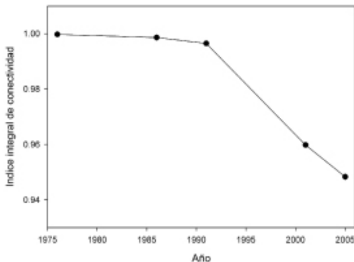
Figura 7. Índice integral de conectividad en Bañados de Iiso para los años 1986, 1991, 2001 y 2005.
