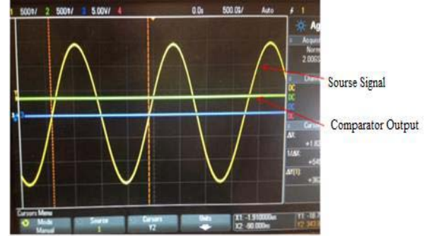
Fig. 19. Output Profile 2.
