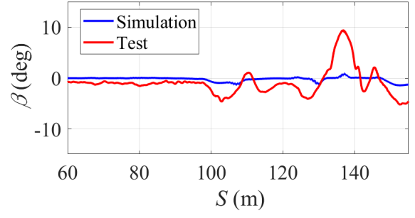
Fig. 10. Side slip angle
