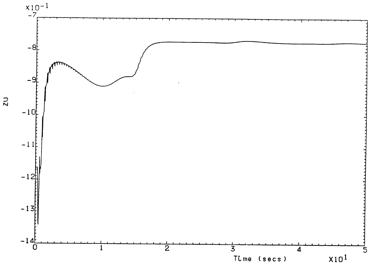
Fig. PI.1-12 z_u estimate (multistep input)
