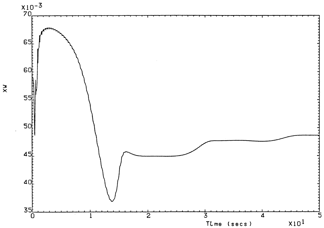
Fig. PI.1-11 x_w estimate (multistep input)
