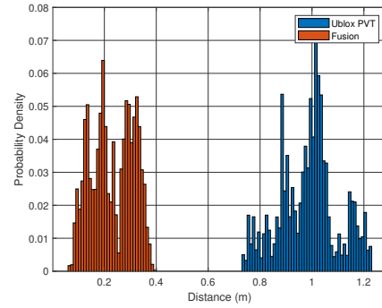
(d) Histogram of distance comparing to RTK
