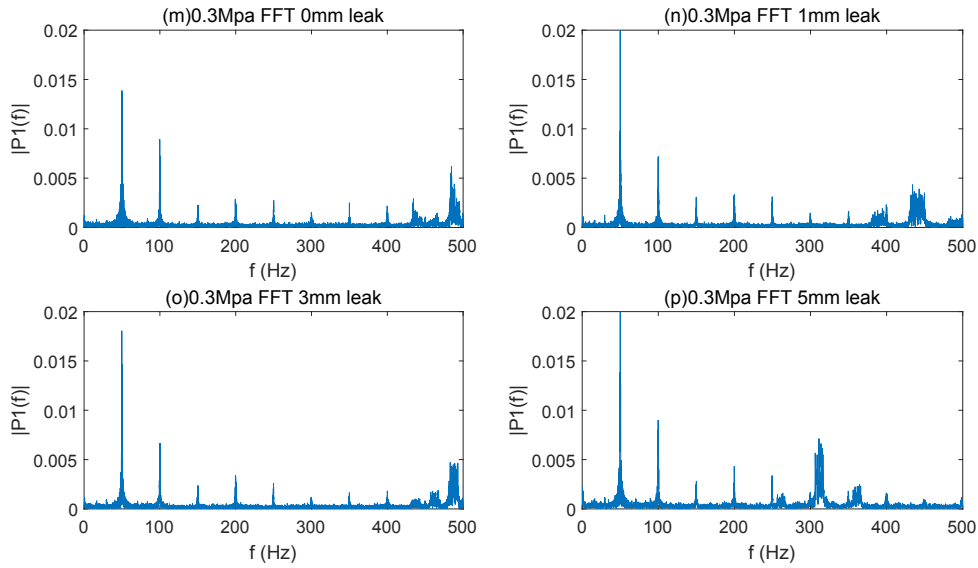
Fig. 14 DPT 1, FFT (1m/s) : (a) 0.10MPa, no leak; (b) 0.10MPa, 1mm; (c) 0.10MPa, 3mm; (d) 0.10MPa, 5mm; (e) 0.20MPa, no leak; (f) 0.20MPa, 1mm; (g) 0.20MPa, 3mm; (l) 0.20MPa, 5mm; (m) 0.30MPa, no leak; (n) 0.30MPa, 1mm; (o) 0.30MPa, 3mm; (p) 0.30MPa, 5mm.
