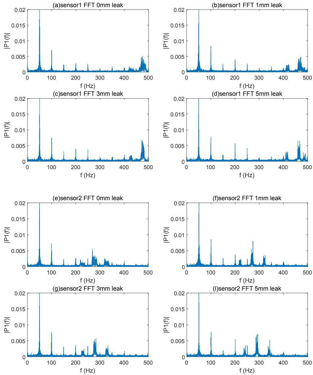
Fig. 12 DPT 1 and DPT 2, FFT (0.20MPa, 1m/s). (a) DPT 1, no leak; (b) DPT 1,1mm; (c) DPT 1,3mm; (d) DPT 1,5mm; (e) DPT 2, no leak; (f) DPT 2,1mm; (g) DPT 2,3mm; (o) DPT 2,5mm.
