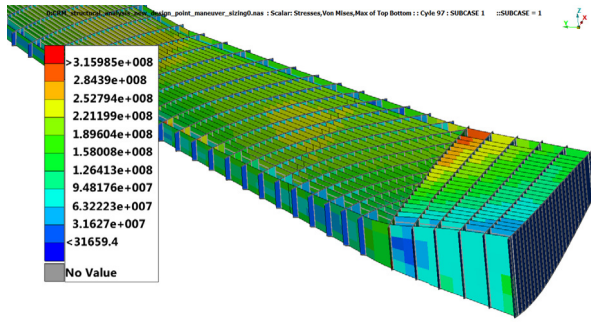
(a) Datum, max Von Mises stress: 315 MPa
