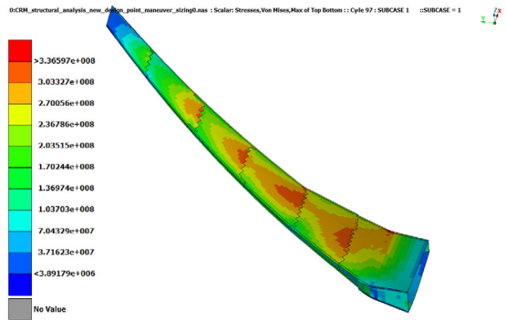
(e) Datum, max Von Mises stress: 315 MPa
