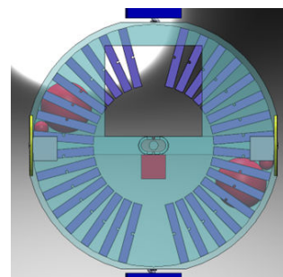
Fig. 16. Tile configuration inside the SV.
