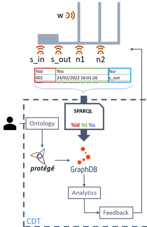
Fig. 14. Data flow in the CDT.
