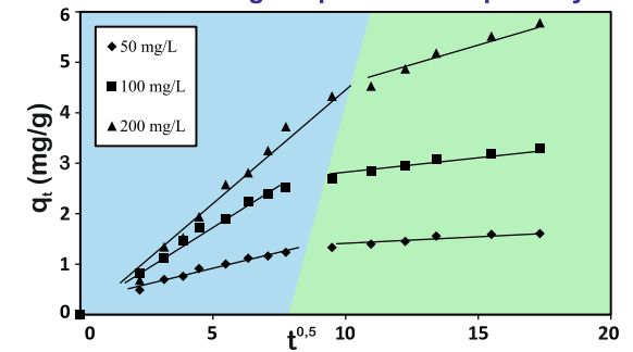
Intraparticle diffusion kinetic model
