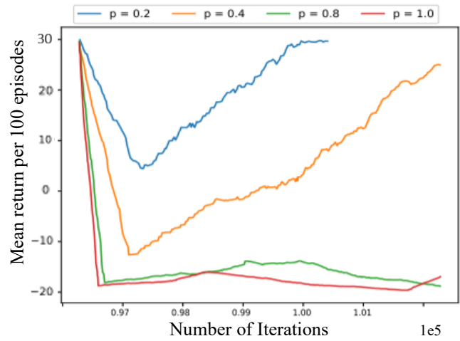
(b) A-PPO
