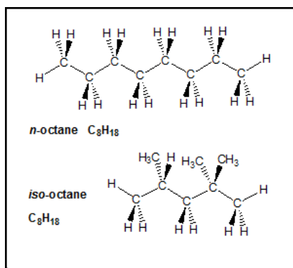
(a) Paraffins
