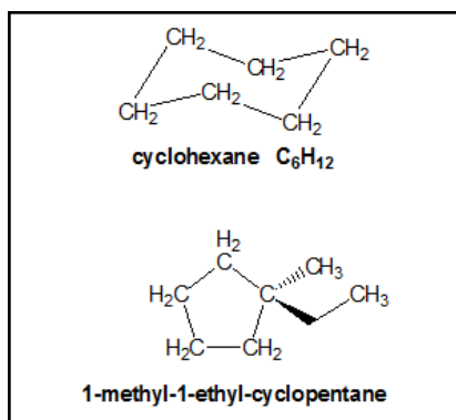
(b) Naphthenes
