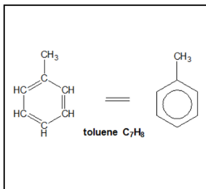
(d) Aromatics
