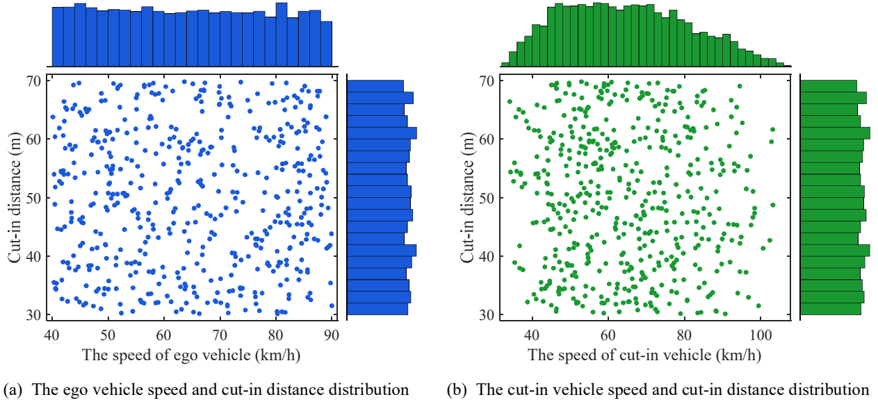
Fig. 12. Parameter distribution of random cut-in scenarios.
