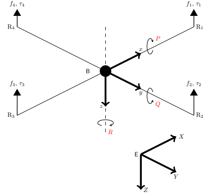
Fig. 2. Quadrotor schematic
