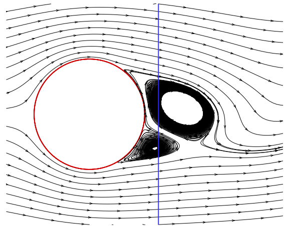
(d) Streamlines – downstream rake.
