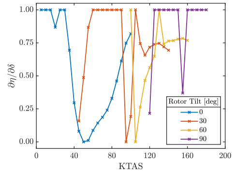
(d) Elevator gearing for the OPSF case
