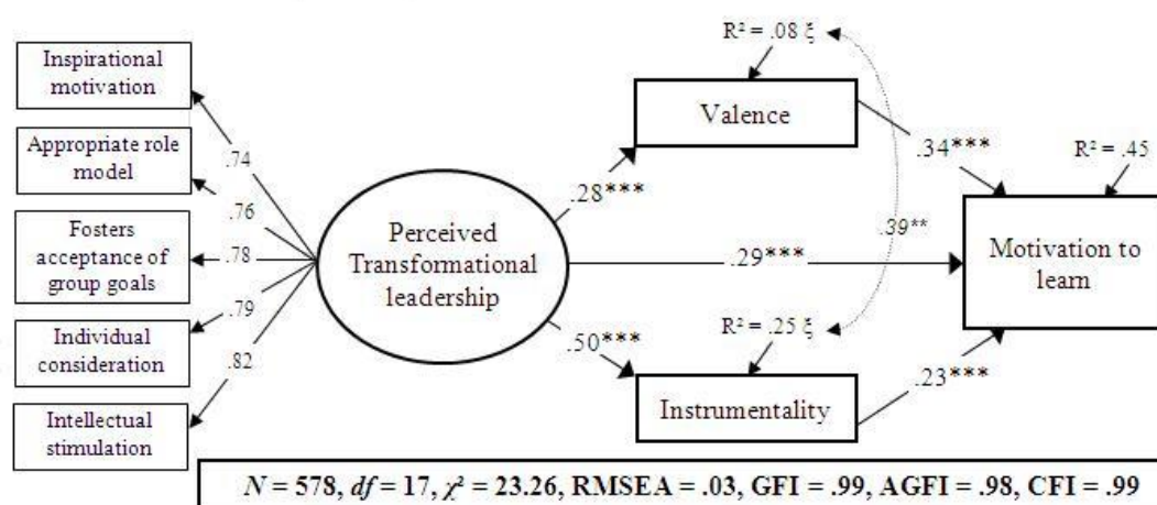
Figure 1. Estimation du maximum de vraisemblance du modèle théorique Maximum likelihood estimation of the theoretical model
