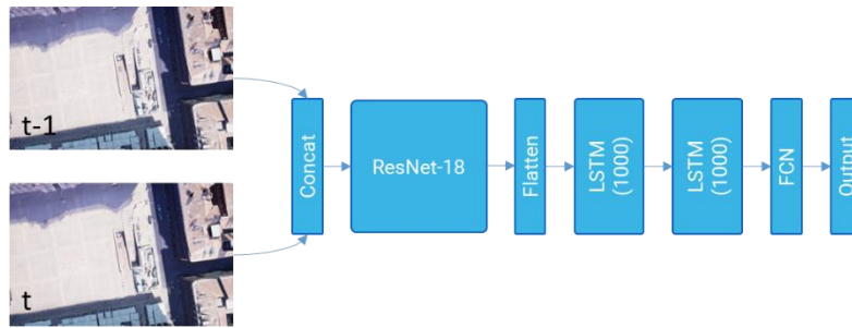
Figure 8: CNN-LSTM VO
