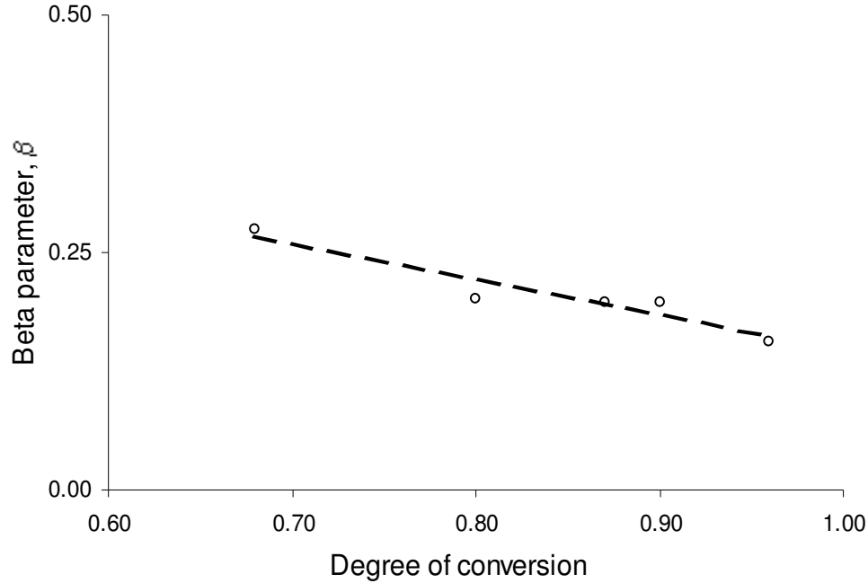
Figure 5 - Linear fitting of the beta parameter values
