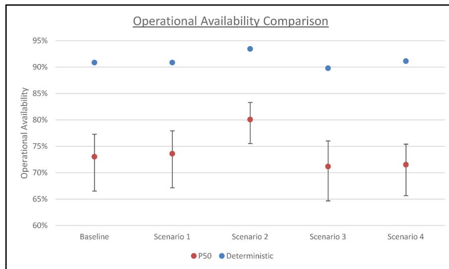
Fig. 7. A_o comparison.
