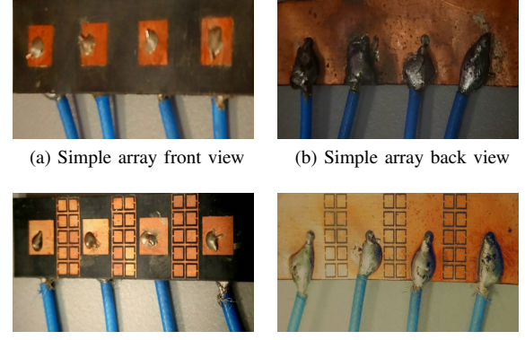
(c) CSRRs loaded array front view (d) CSRRs loaded array back view
