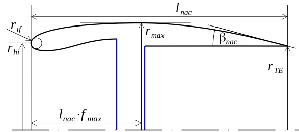
Fig. 3. The parameters used to specify the nacelle geometry.
