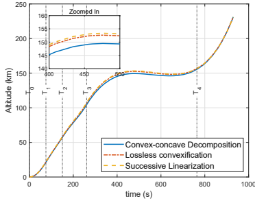
(f) Altitude
