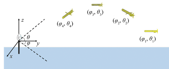
Fig. 11. Radar detection scenario.
