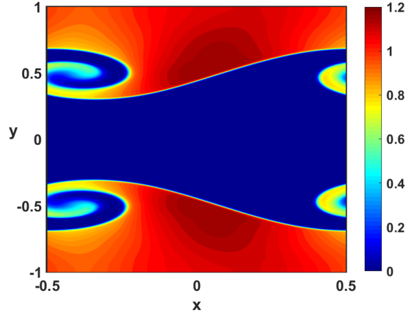
(b) 1024 \times 2048 : MUSCL2
