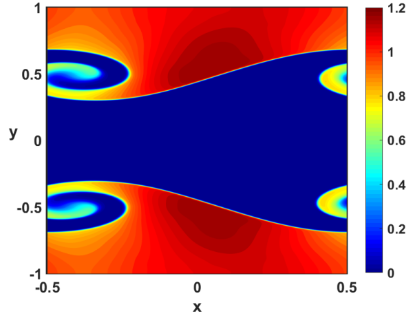
(d) 1024 \times 2048 : WENO3
